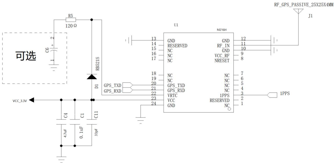
图 6：无源天线通用参考设计
