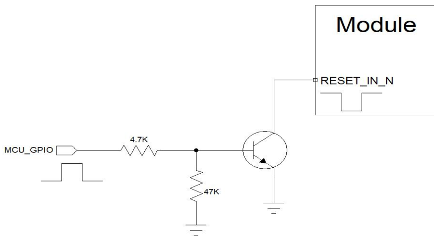
图 2：复位接口参考设计
