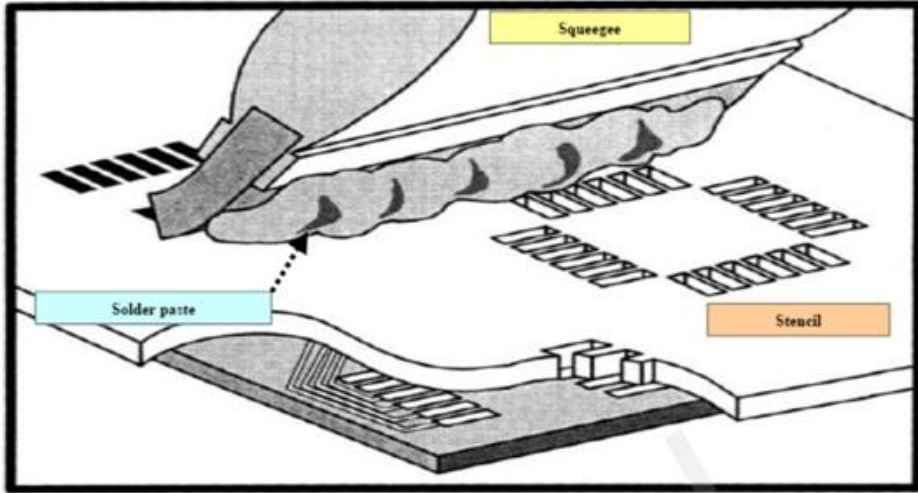
图 11：印膏图
