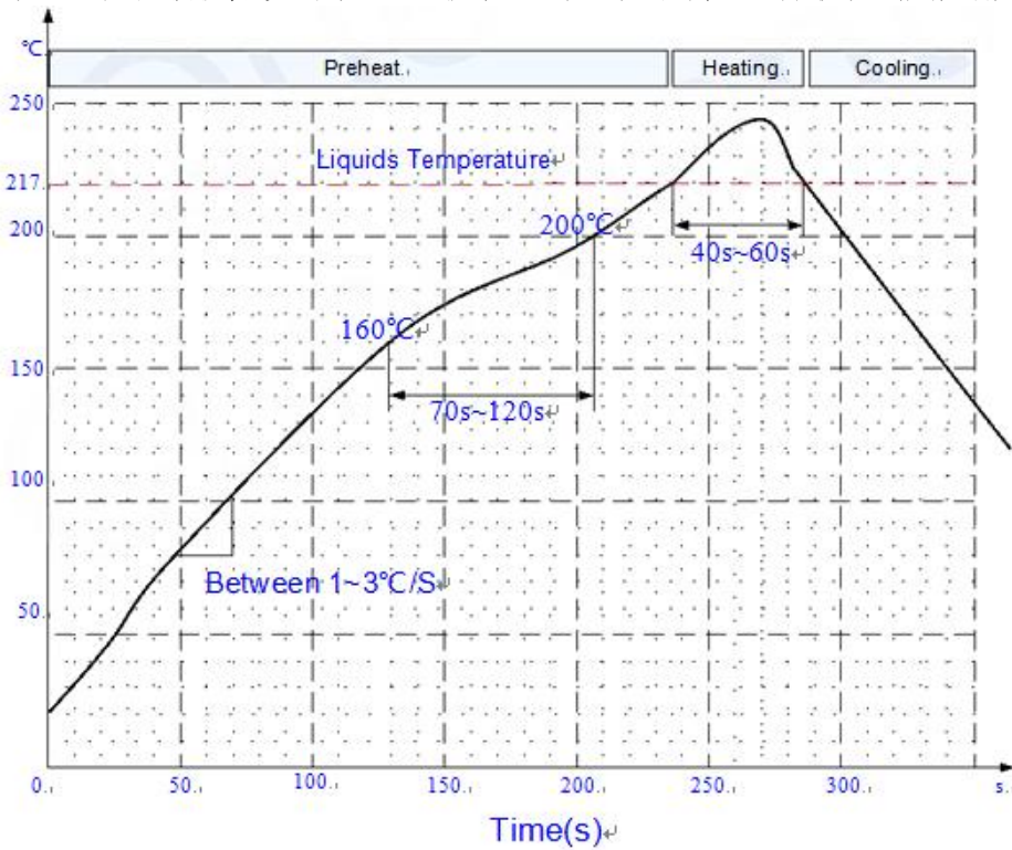
图 12：炉温曲线
