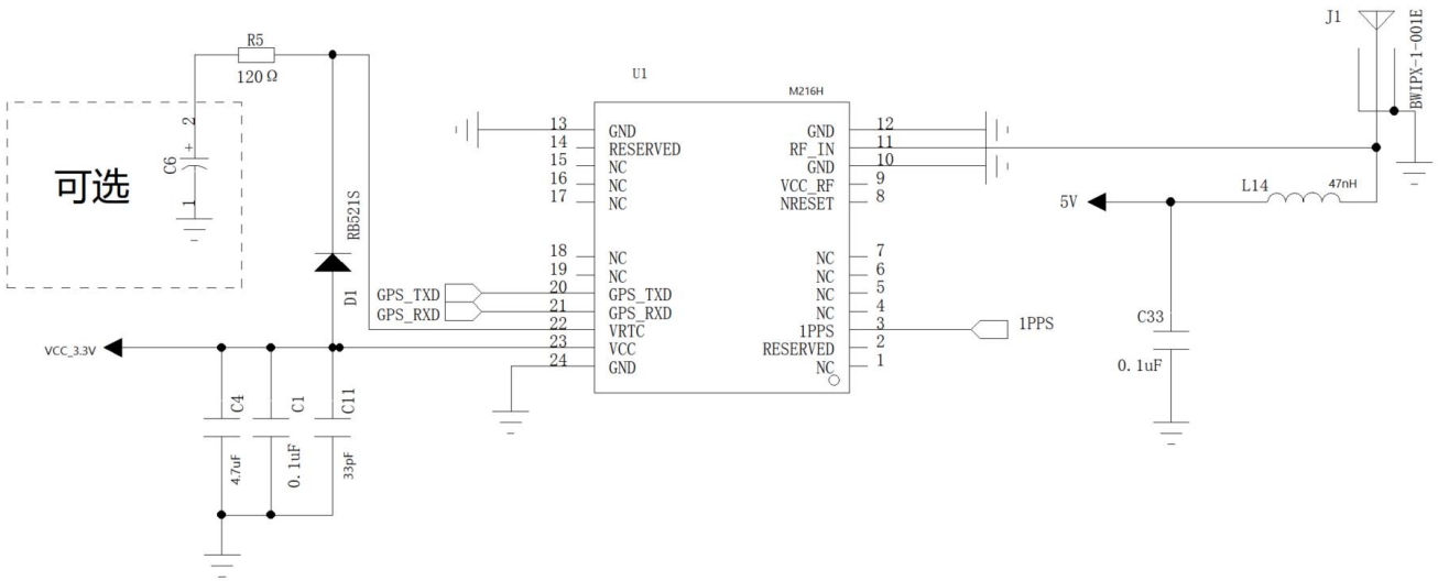
图 6: 5V 有源天线参考设计
