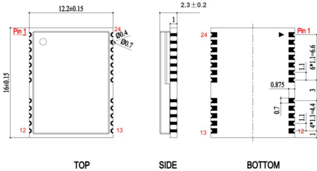
图 8: M216H 尺寸图 (单位: 毫米)
