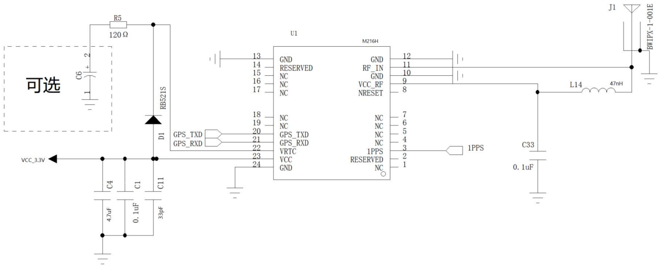
图 5: 3.3V 有源天线参考设计
