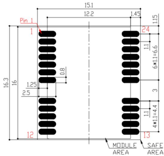
图 9: 正视图, M216H PCB 封装 (单位: 毫米)
